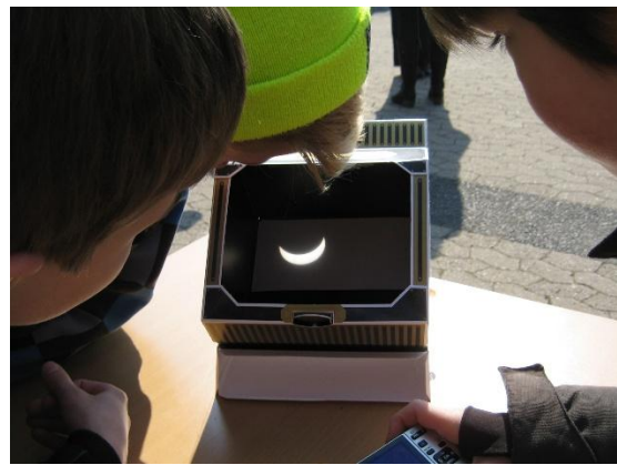
Physikübung: partielle Sonnenfinsternis
