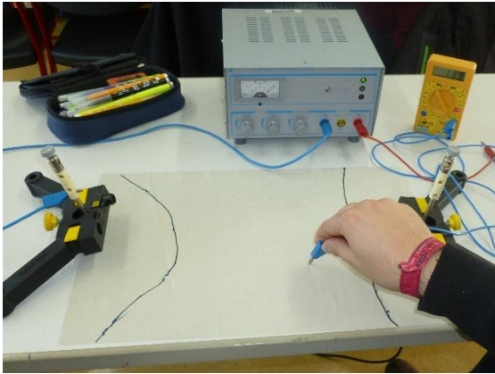
Physikübung: Äquipotentiallinien
